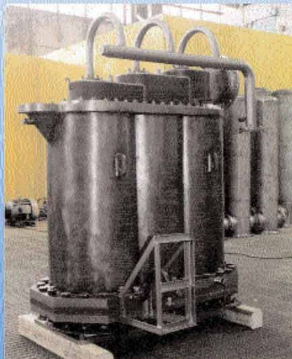
Эжактор ЭПО 3-75/25
